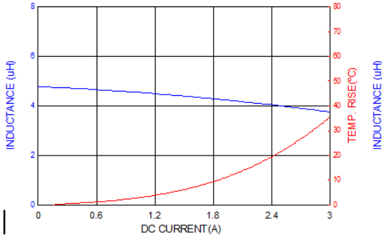
PICQ0412HP4R7MF
