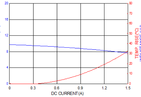
PICQ0412HP100MF
