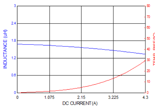
PICQ0412HP1R5MF
