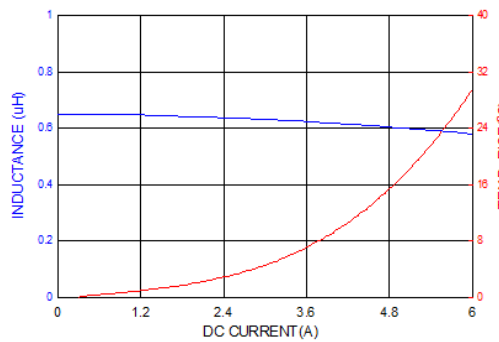
PICQ0412HPR68MF
