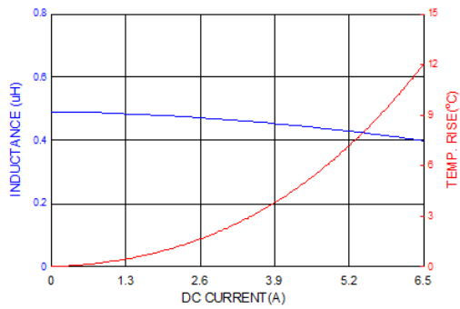
PICQ0412HPR47MF
