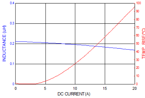
PICQ0412HPR22MF
