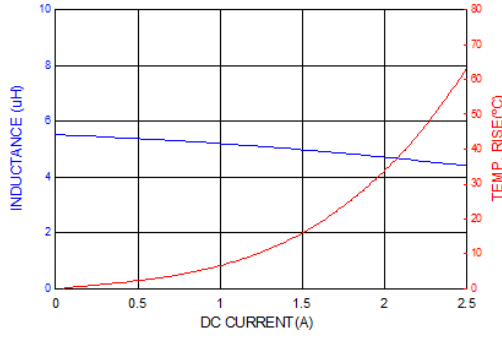
PICQ0412HP5R6MF
