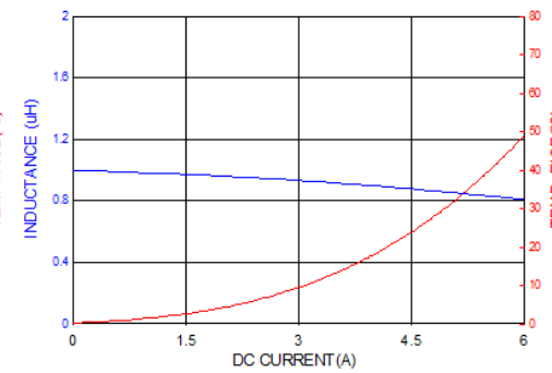
PICQ0412HP1R0MF
