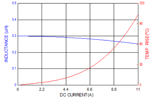
PICQ0412HPR33MF
