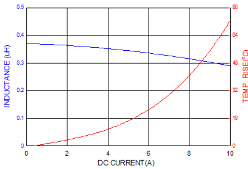
PICQ0412HPR36MF
