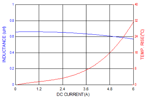
PICQ0412HPR60MF
