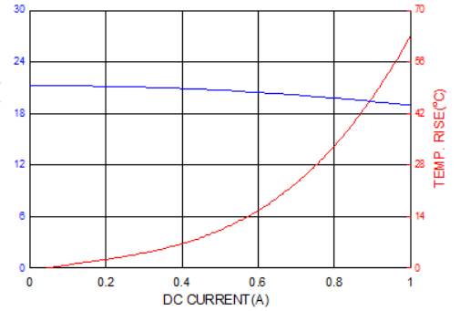
PICQ0412HP220MF
