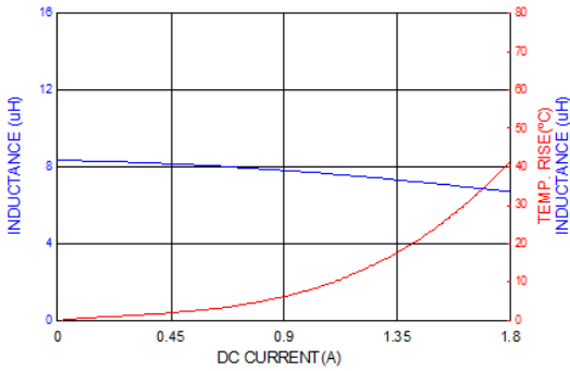
PICQ0412HP8R2MF
