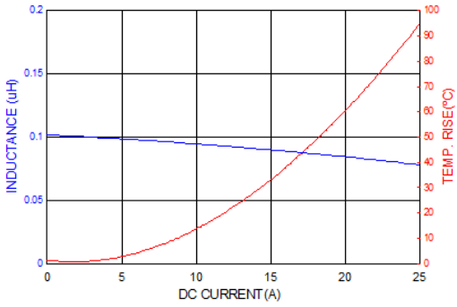
PICQ0412HPR10YF
