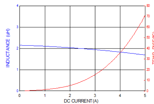
PICQ0412HP2R2MF
