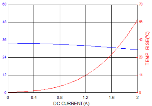
PICQ0503H330MF
