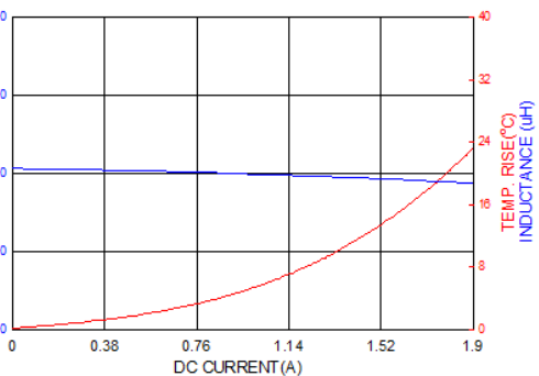
PICQ0503H220MF
