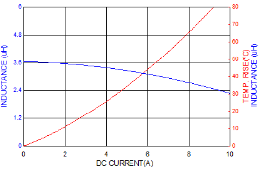
PICQ0503H3R6MF
