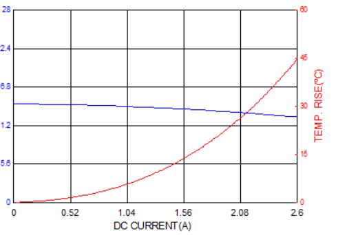
PICQ0503H150MF
