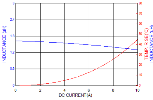
PICQ0503H1R5MF
