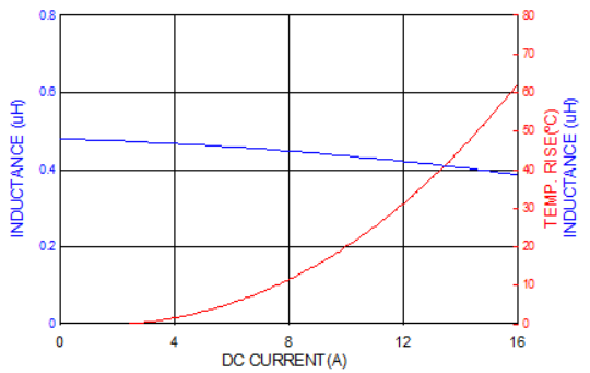
PICQ0503HR47MF
