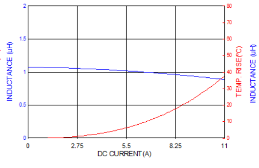
PICQ0503H1R0MF
