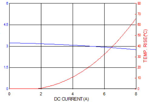
PICQ0503H5R6MF
