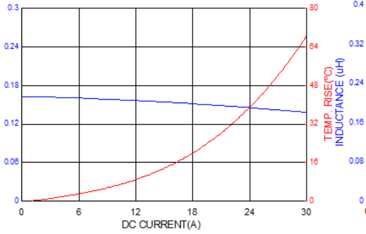
PICQ0503HR15YF
