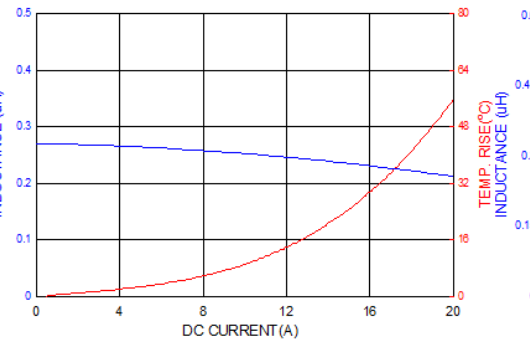
PICQ0503HR25MF
