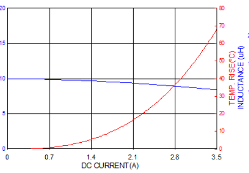
PICQ0503H100MF
