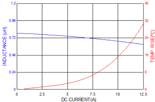
PICQ0503HR82MF
