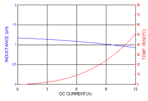
PICQ0503H1R2MF
