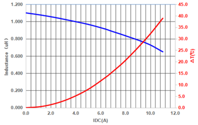
PIF0403LR1R0MN
