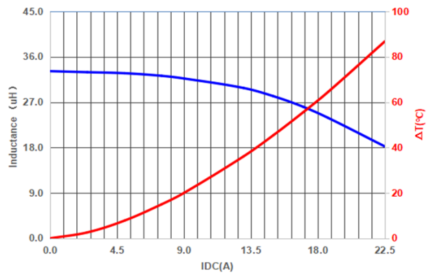
PIFQ1510A330MO
