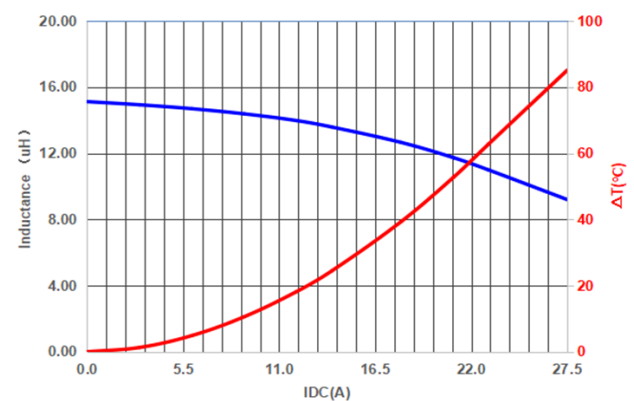
PIFQ1510A150MO
