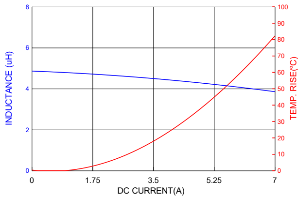
PIC0618H4R7MF
