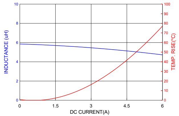
PIC0618H5R6MF
