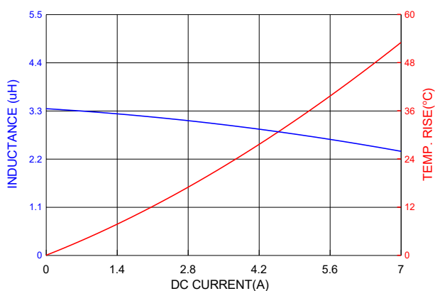
PIAQ0502SP3R3MN
