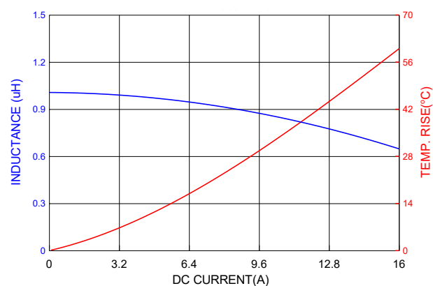
PIAQ0602S1R0MN
