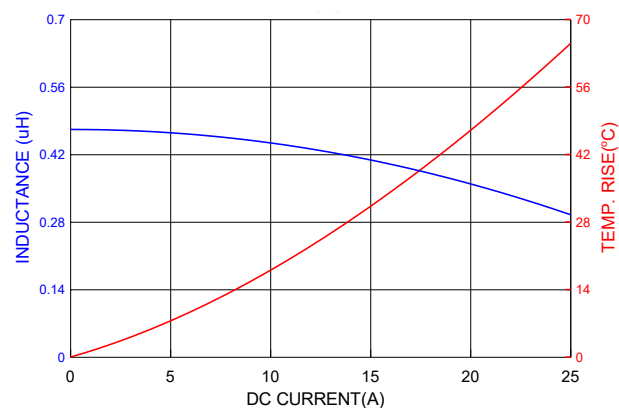
PIAQ0602SR47MN
