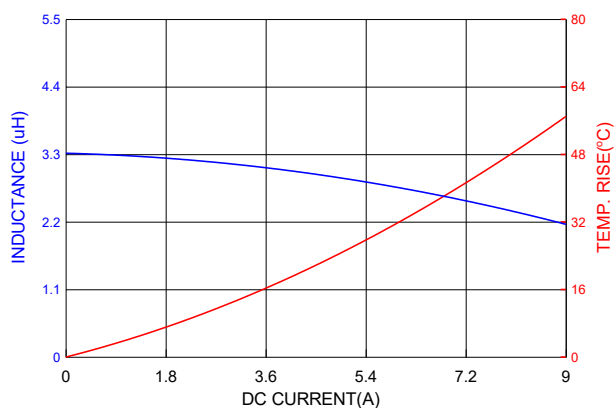
PIAQ0602S3R3MN
