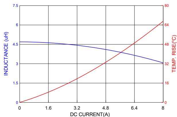
PIAQ0602S4R7MN
