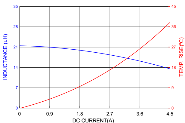
PIAQ0605S220MN
