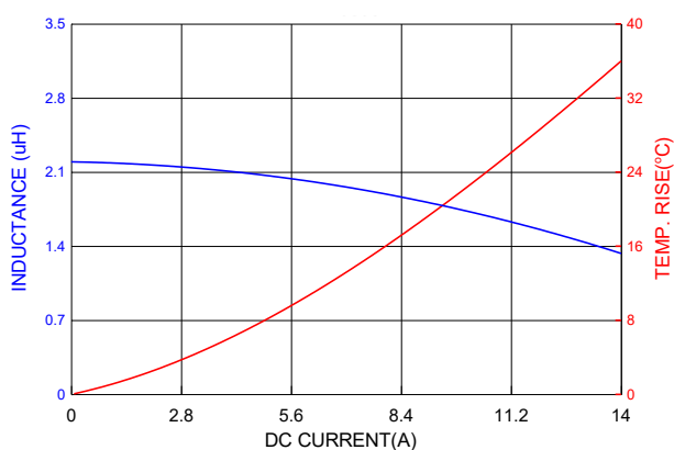
PIAQ0605S2R2MN
