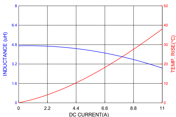
PIAQ0605S4R7MN
