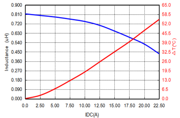
PIAQ0605SR82MN
