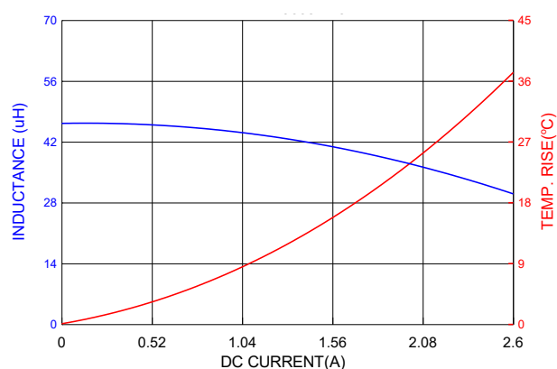
PIAQ0605S470MN
