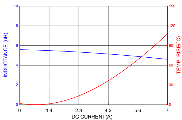
PICQ0503HP5R6MF
