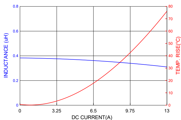
PICQ0512HPR36MF
