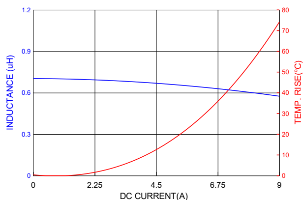
PICQ0512HPR68MF
