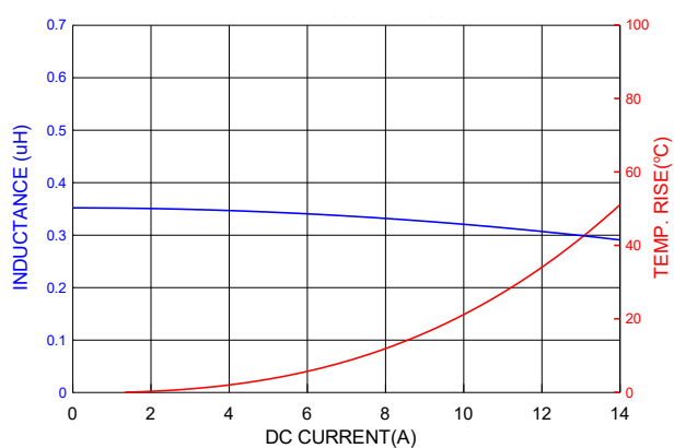
PICQ0512HPR33MF
