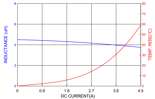
PICQ0518HP4R7MF
