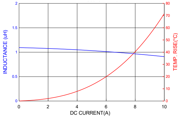
PICQ0518HP1R0MF
