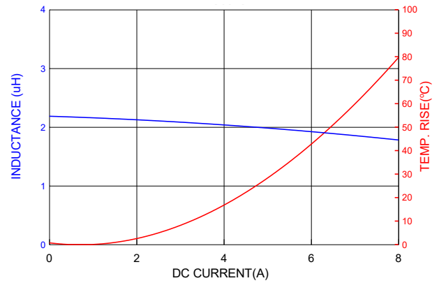
PICQ0518HP2R2MF
