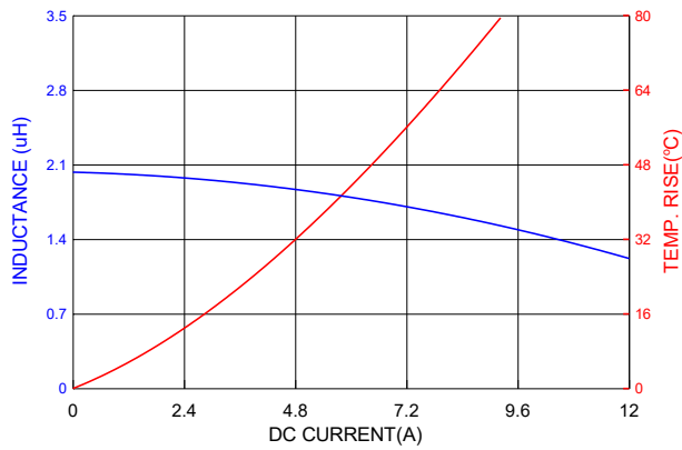
PICQ0518HP2R0MF
