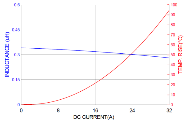
PICQ0603HR36MF
