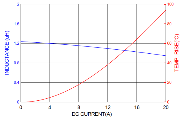
PICQ0603H1R2MF
