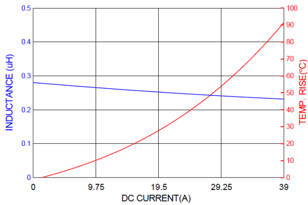
PICQ0603HR25MF
