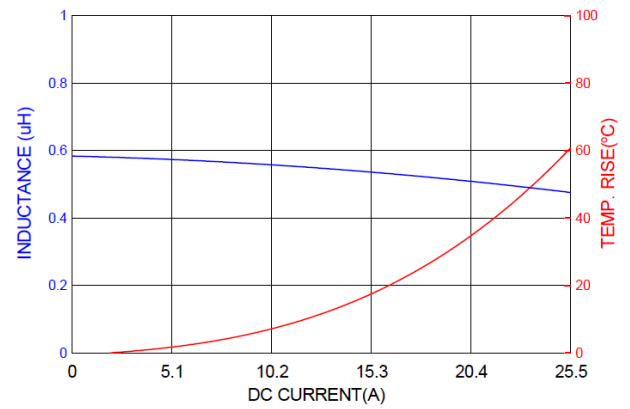
PICQ0603HR60MF
