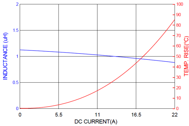
PICQ0603H1R0MF
