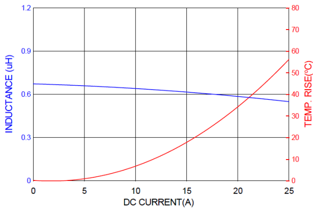
PICQ0603HR68MF
