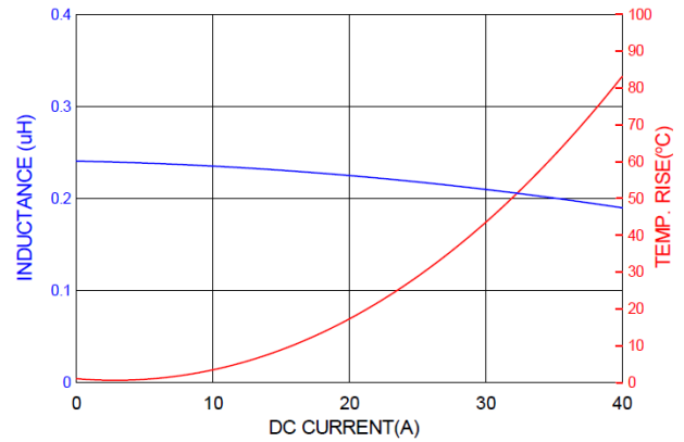
PICQ0603HR22YF
