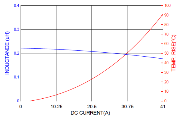
PICQ0603HR19YF
