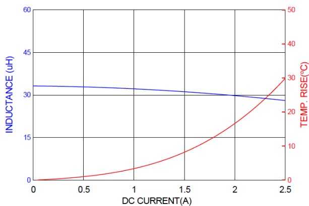
PICQ0603H330MF
