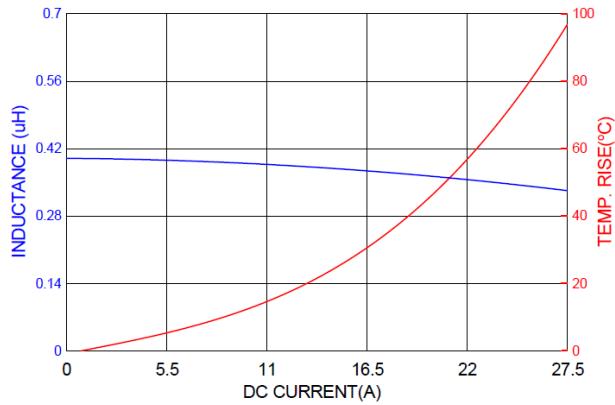
PICQ0603HR40MF
