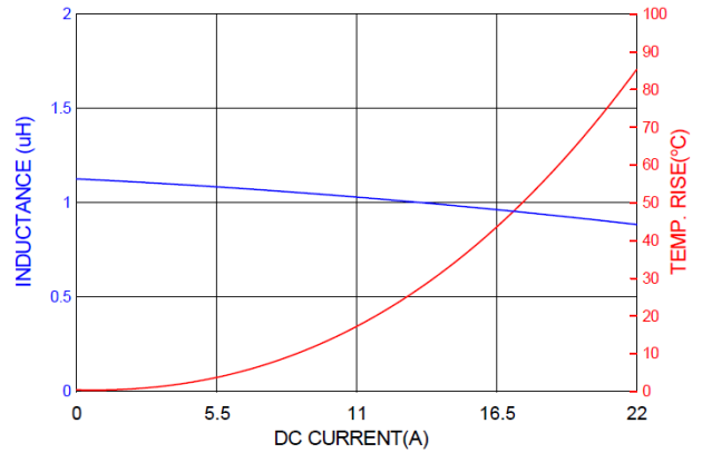
PICQ0603HR90MF
