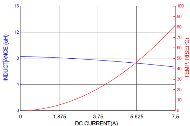
PICQ0603H8R2MF
