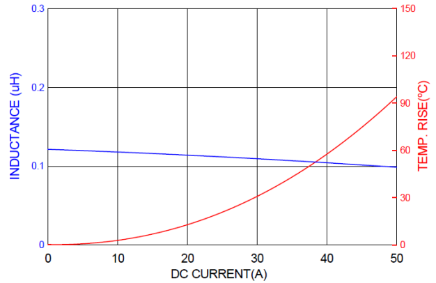
PICQ0603HR13YF
