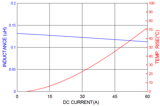
PICQ0603HR10YF
