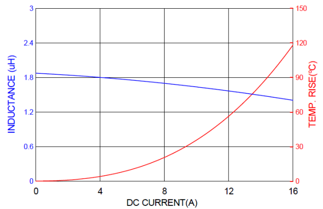
PICQ0603H1R8MF
