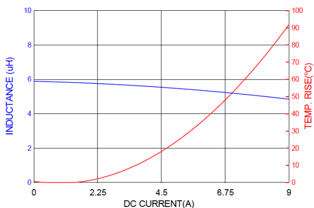
PICQ0603H5R6MF
