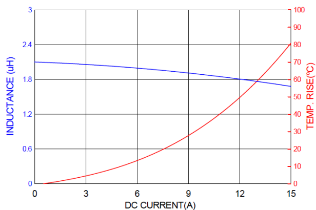
PICQ0603H2R0MF
