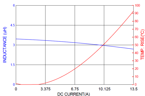
PICQ0603H3R3MF
