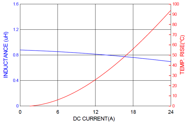
PICQ0603HR82MF
