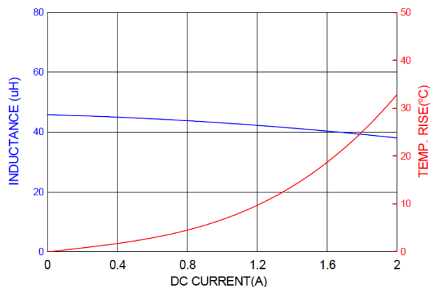
PICQ0603H470MF
