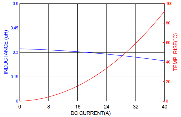
PICQ0603HR30MF
