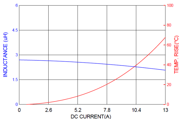
PICQ0603H2R7MF
