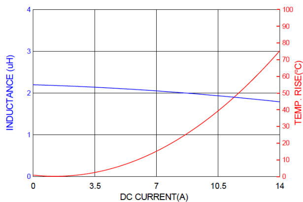
PICQ0603H2R2MF
