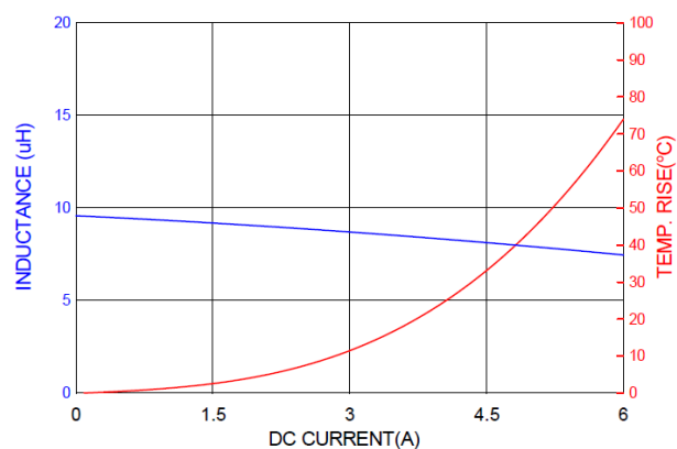
PICQ0603H100MF
