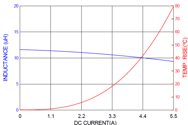
PICQ0603H120MF
