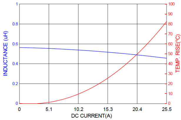
PICQ0603HR56MF
