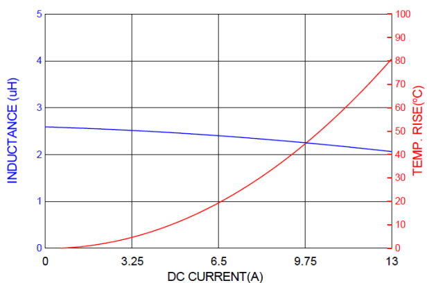
PICQ0603H2R5MF
