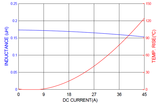
PICQ0603HR16YF
