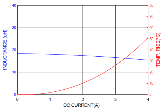
PICQ0603H180MF
