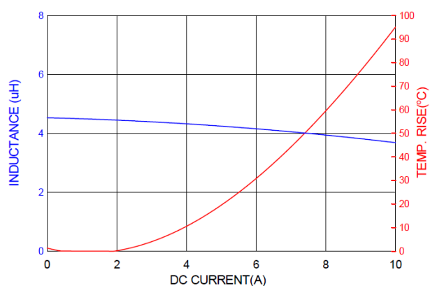
PICQ0603H4R7MF
