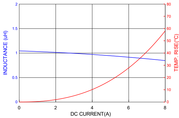
PICQ0612H1R0MF
