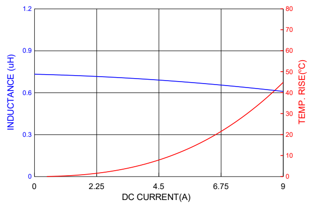
PICQ0612HR68MF
