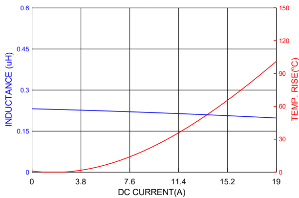
PICQ0612HR22YF
