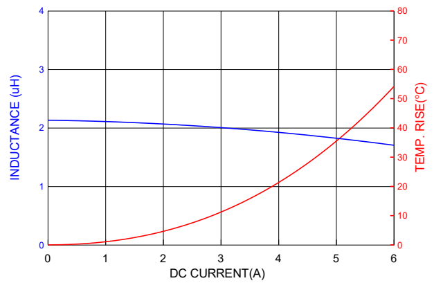
PICQ0612H2R2MF
