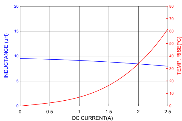
PICQ0612H100MF
