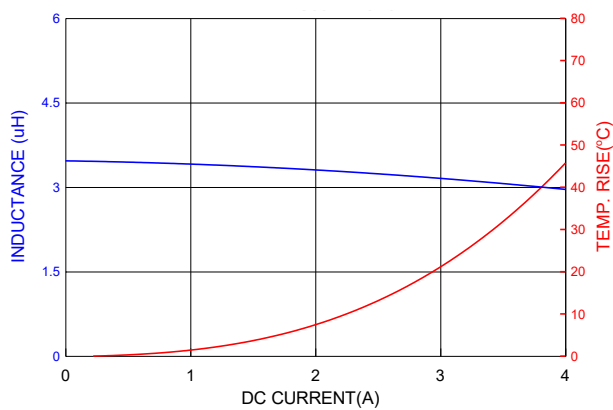
PICQ0612H3R3MF
