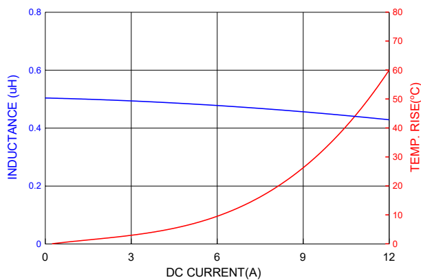
PICQ0612HR47MF
