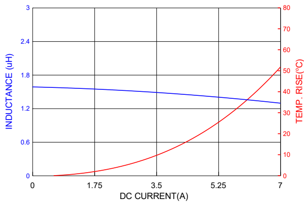
PICQ0612H1R5MF
