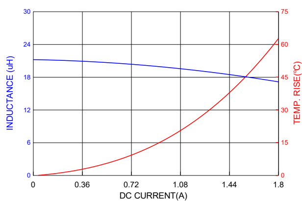
PICQ0612H220MF
