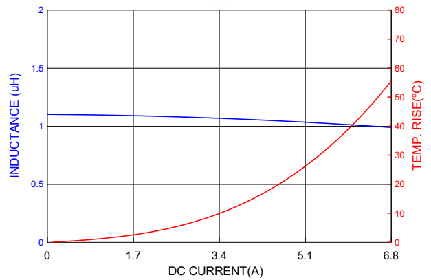
PICQ0612H1R2MF
