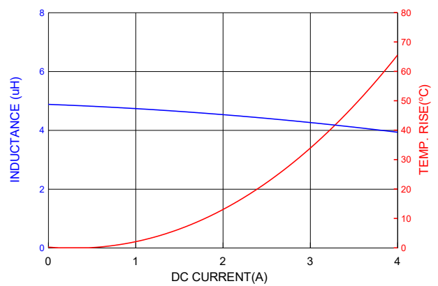
PICQ0612H4R7MF
