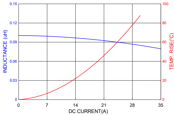
PICQ0612HR10YF
