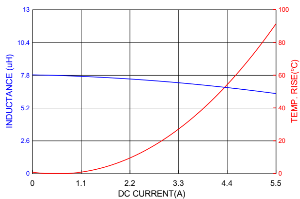
PICQ0624H8R2MF
