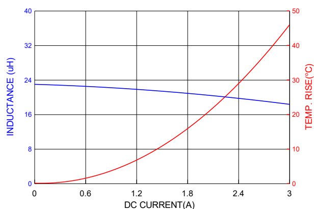
PICQ0624H220MF
