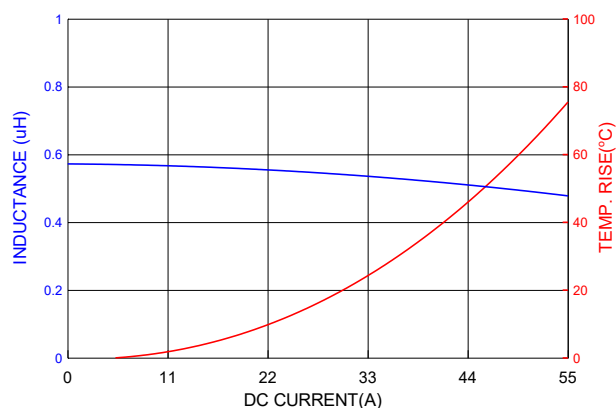
PICQ1205HPR56MF
