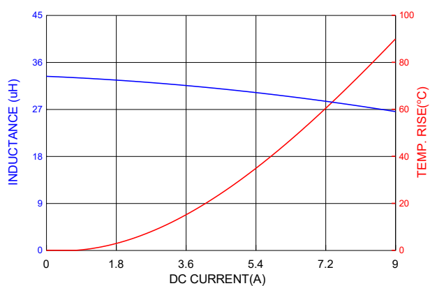
PICQ1205HP330MF
