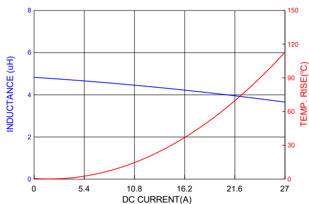
PICQ1205HP4R7MF
