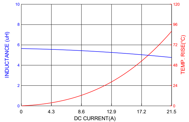
PICQ1205HP6R0MF
