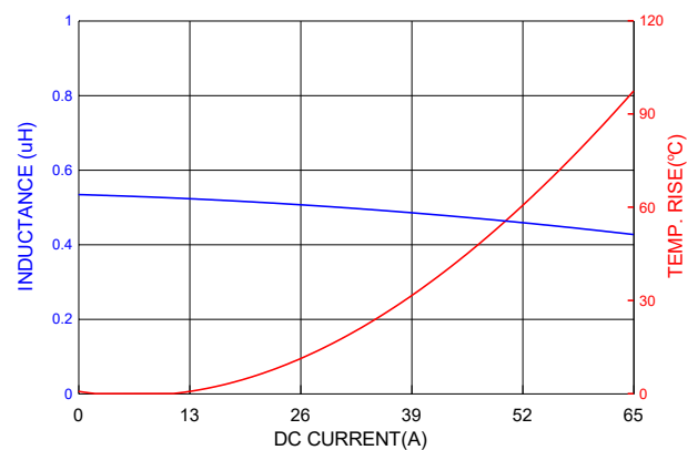
PICQ1205HPR47MF
