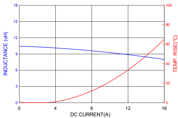
PICQ1205HP100MF
