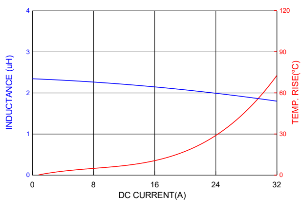
PICQ1205HP2R2MF
