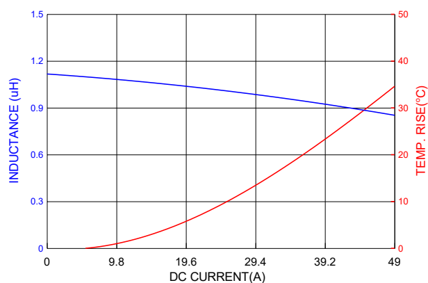
PICQ1205HP1R2MF
