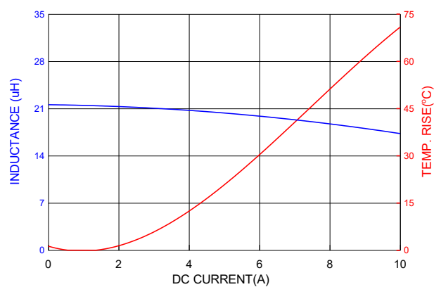
PICQ1205HP220MF
