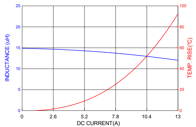
PICQ1205HP150MF
