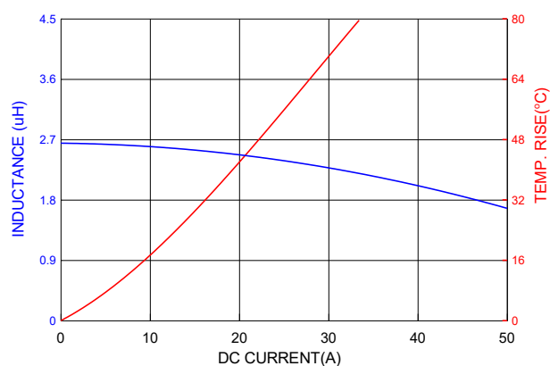
PICQ1205HP2R7MF
