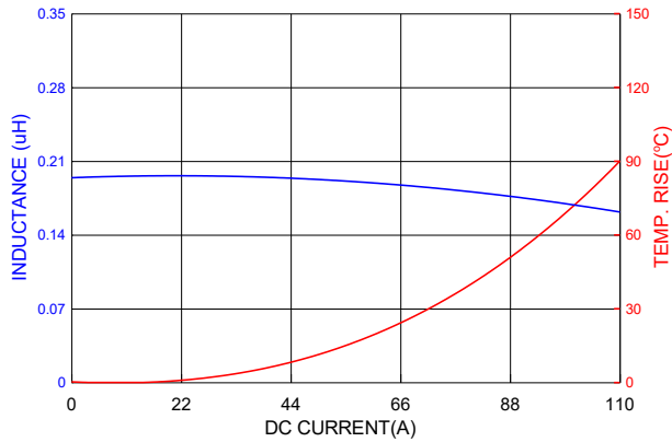
PICQ1205HPR20MF
