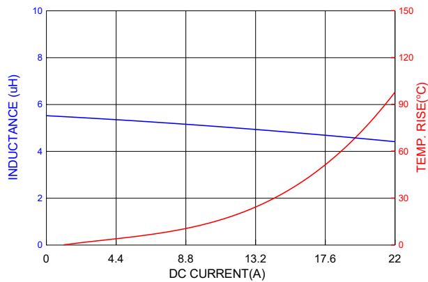
PICQ1205HP5R6MF
