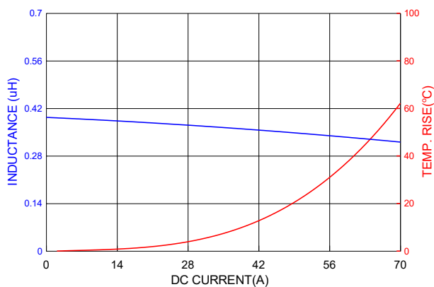
PICQ1205HPR39MF
