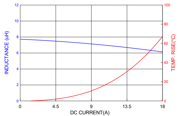
PICQ1205HP8R2MF
