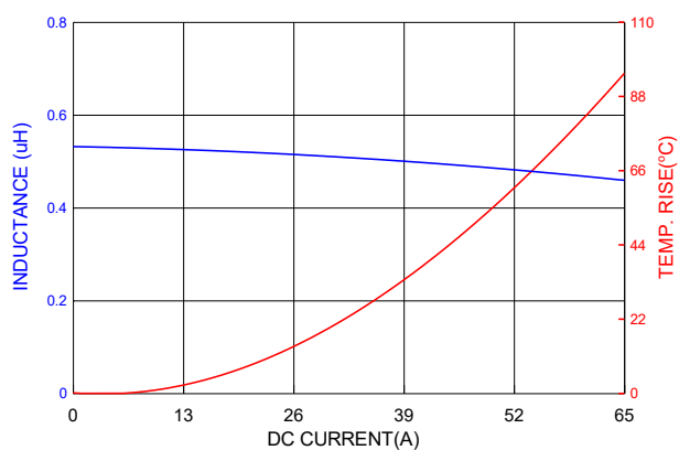
PICQ1205HPR50MF
