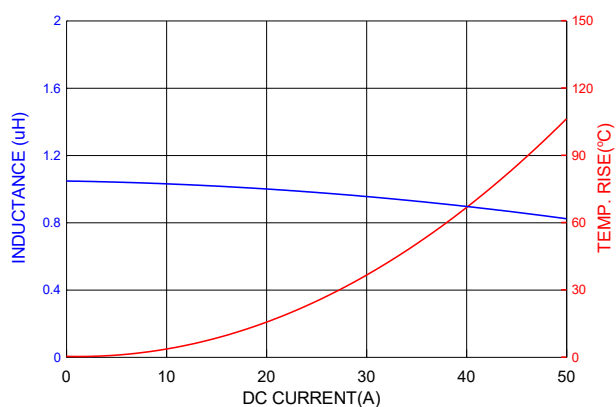
PICQ1205HP1R0MF
