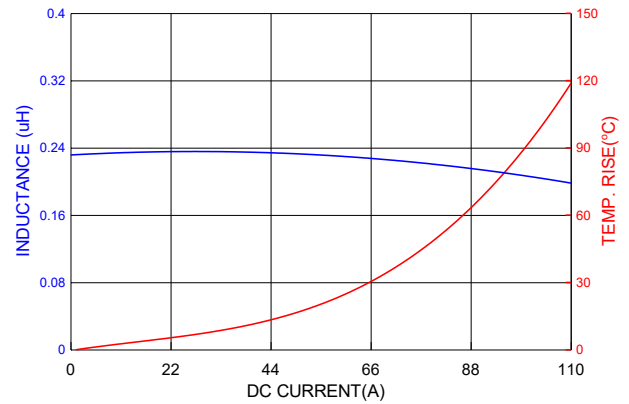
PICQ1205HPR22MF
