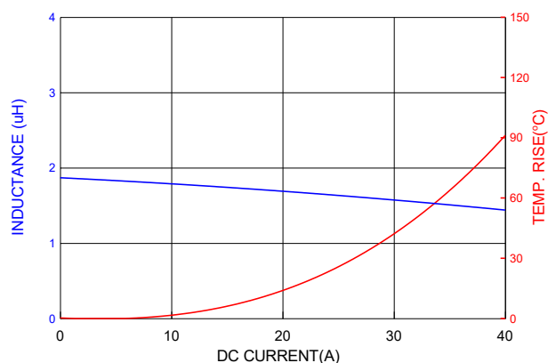
PICQ1205HP1R8MF
