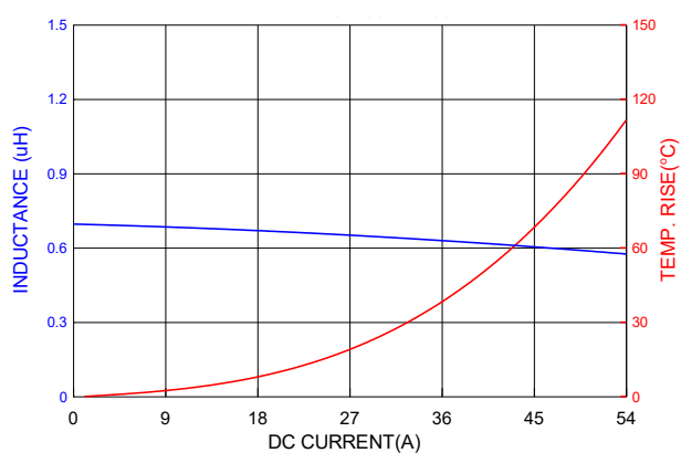
PICQ1205HPR68MF
