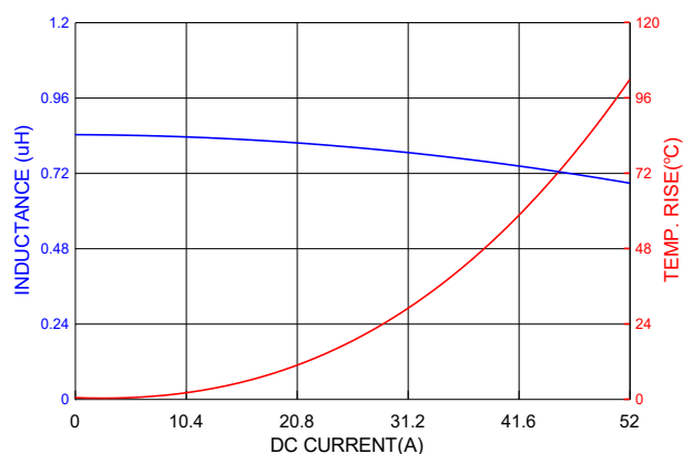
PICQ1205HPR82MF
