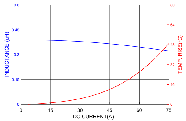
PICQ1205HPR36MF
