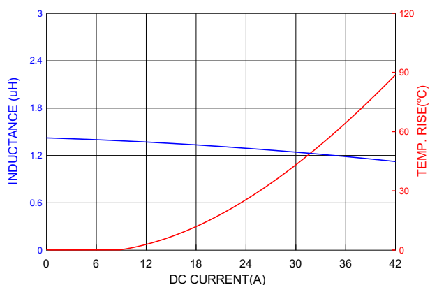
PICQ1205HP1R5MF
