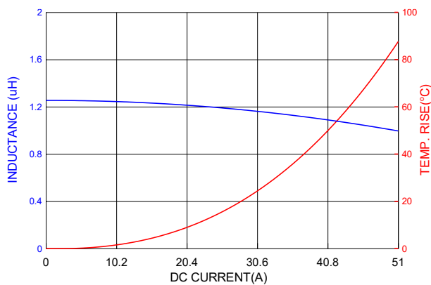
PICQ1206HP1R2MF
