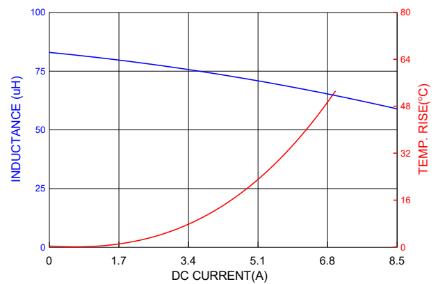
PICQ1206HP820MF
