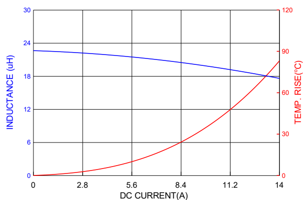
PICQ1206HP220MF
