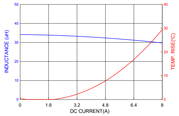
PICQ1206HP330MF
