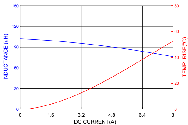
PICQ1206HP101MF
