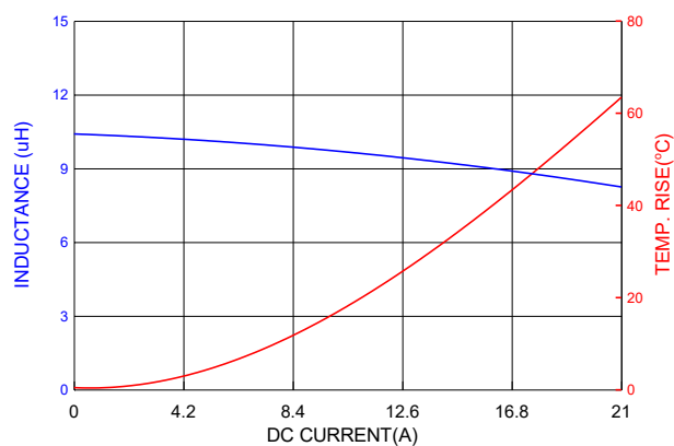
PICQ1206HP100MF
