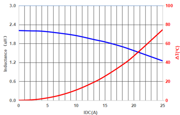
PIFQ0707A2R2MO
