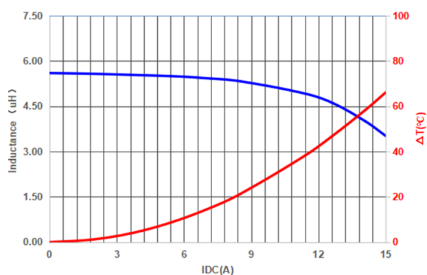
PIFQ0707A5R6MO
