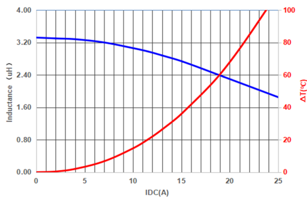
PIFQ0707A3R3MO
