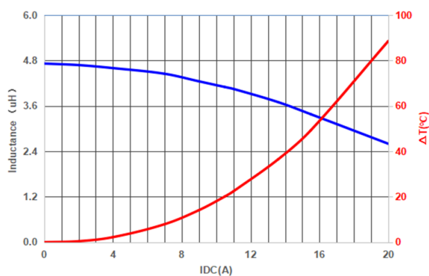
PIFQ0707A4R7MO
