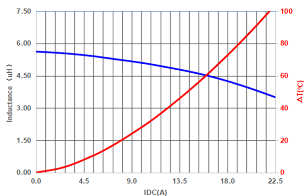
PIFQ1006A5R6MO
