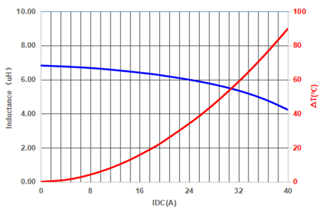
PIFQ1510A6R8MO
