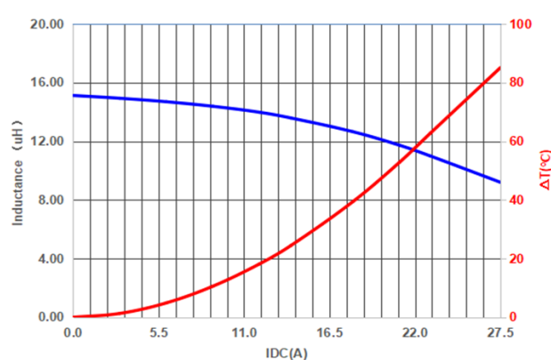
PIFQ1510A150MO
