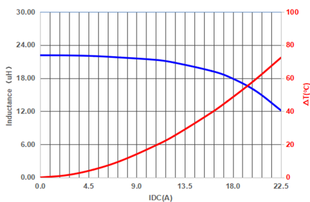
PIFQ1510A220MO
