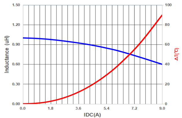
PIMQ322520A1R0MN
