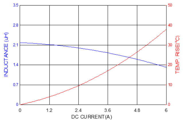
PIA0402SP2R2MN
