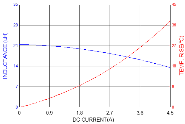
PIA0605S220MN
