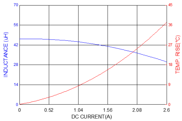
PIA0605S470MN
