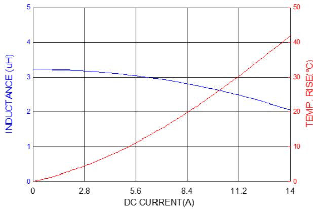
PIA0605S3R3MN
