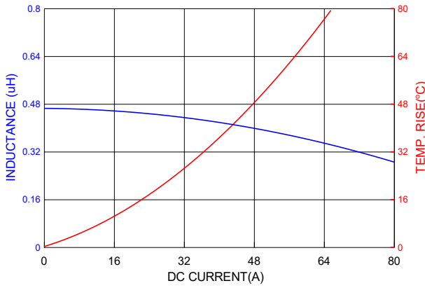
PIA1205SPR47MN
