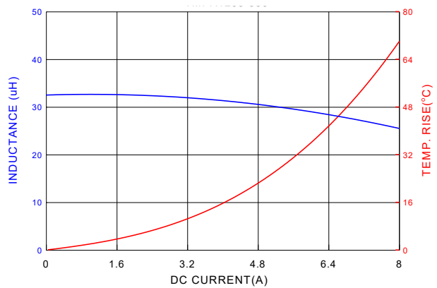
PIA1205SP330MN
