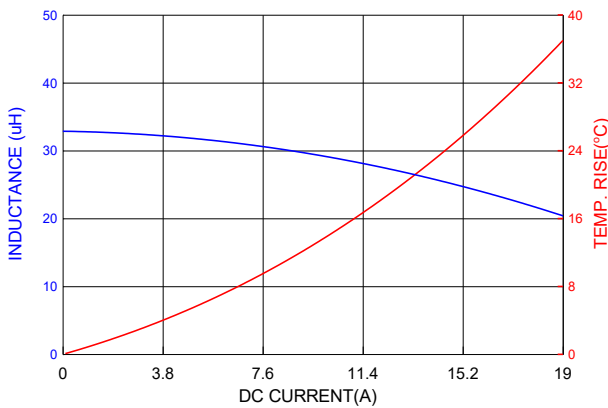
PIA2313SP330MN
