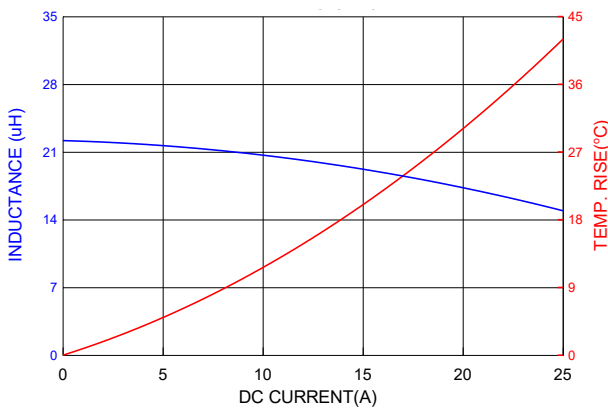
PIA2313SP220MN
