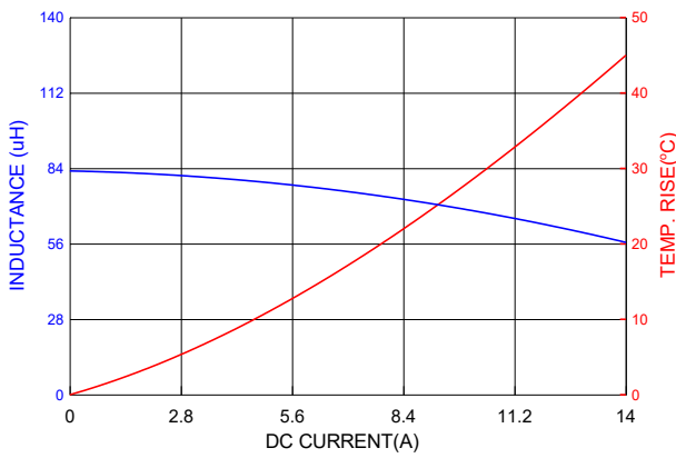
PIA2313SP820MN
