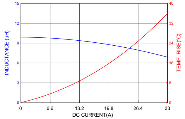
PIA2313SP100MN
