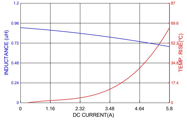
PIC0312HR82MF
