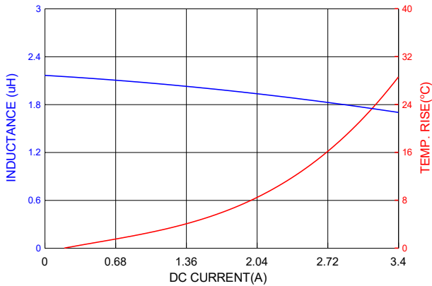
PIC0312H2R2MF
