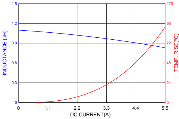
PIC0312H1R0MF
