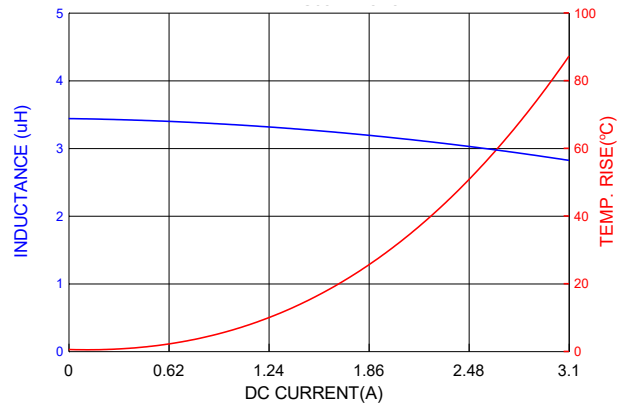
PIC0312H3R3MF
