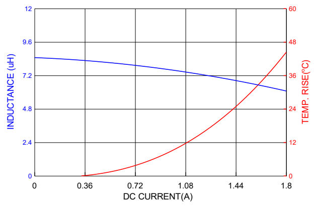
PIC0315H8R2MF
