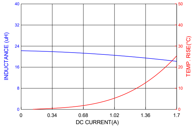
PIC0515HP220MF
