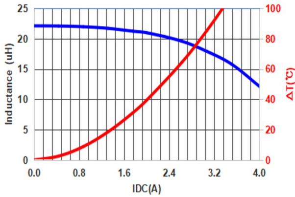
PIC0603H220MF
