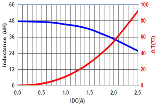
PIC0603H470MF
