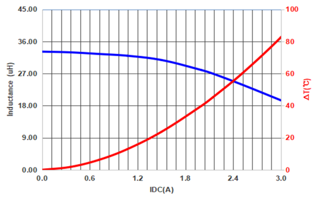
PIC0603H330MF
