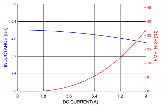
PIC0604H5R6MF
