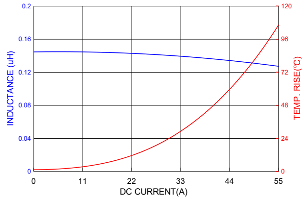
PIC0604HR15YF
