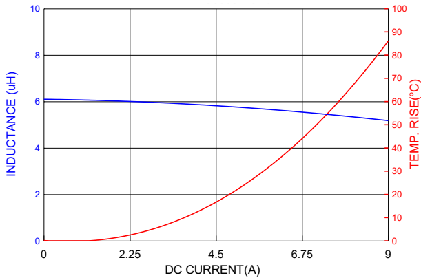
PIC0605H5R6MF
