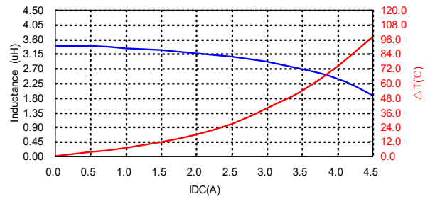
PIC0612H3R3MF
