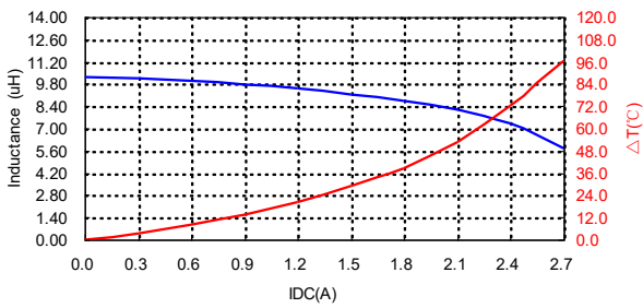
PIC0612H100MF
