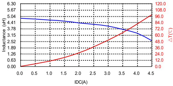
PIC0612H4R7MF
