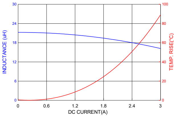
PIC0615H220MF
