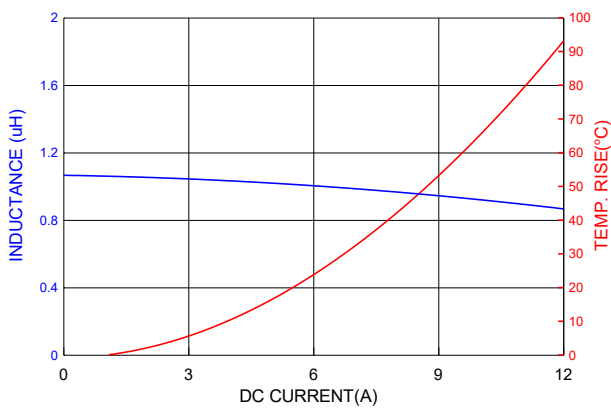
PIC0615H1R0MF
