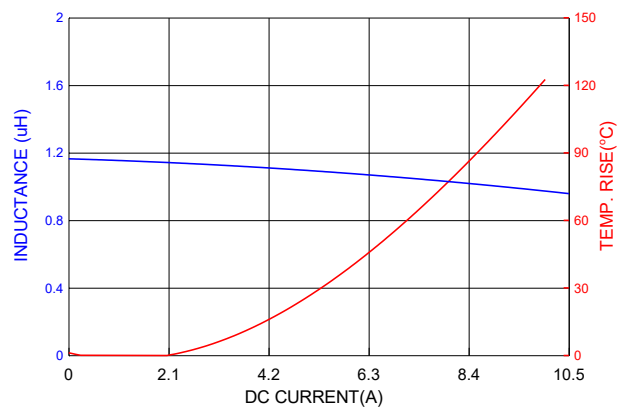
PIC0615H1R2MF
