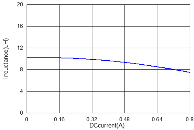
PNS3012T100MF
