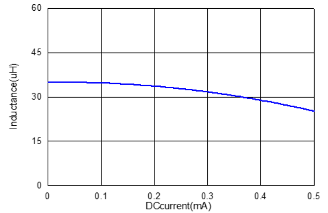
PNS3012T330MF
