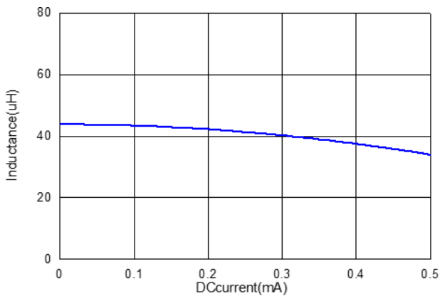
PNS3012T470MF
