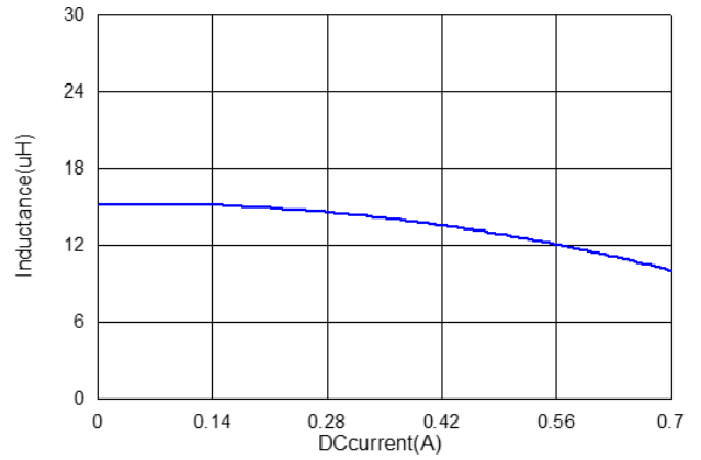
PNS3012T150MF
